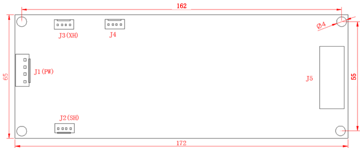
图 2.6 BL2000-HXK-V9 尺寸图 (单位 mm)
