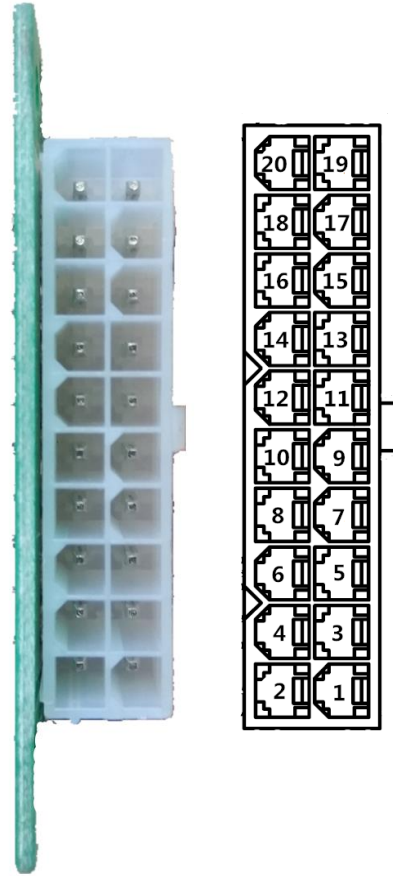
图 2.5 J5 端子序号图
