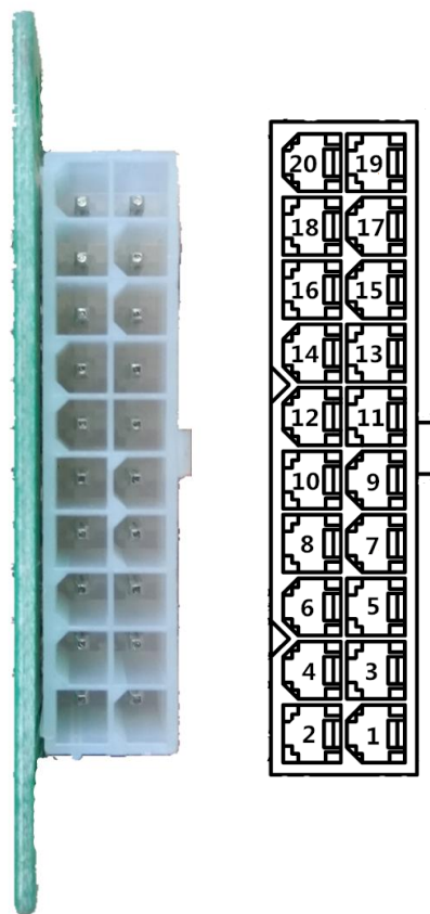
图 2.2 J5 端子序号图
